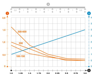
Belastningsdiagram gitterrenne type GRM 105
